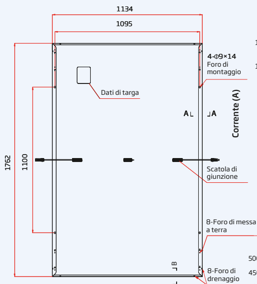
Vista Retro
