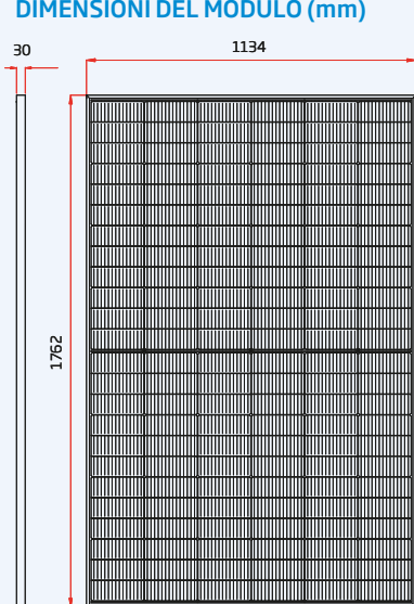
Vista Frontale
